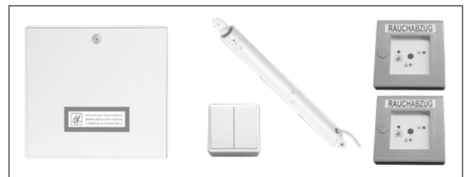
VdS-zertifiziertes Entrauchungsset für Treppenhäuser, zertifiziert nach DIN EN12101-10 und geprüft nach ISO 21627-9.
